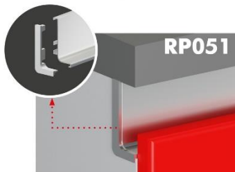
L-образный профиль под столешницу
